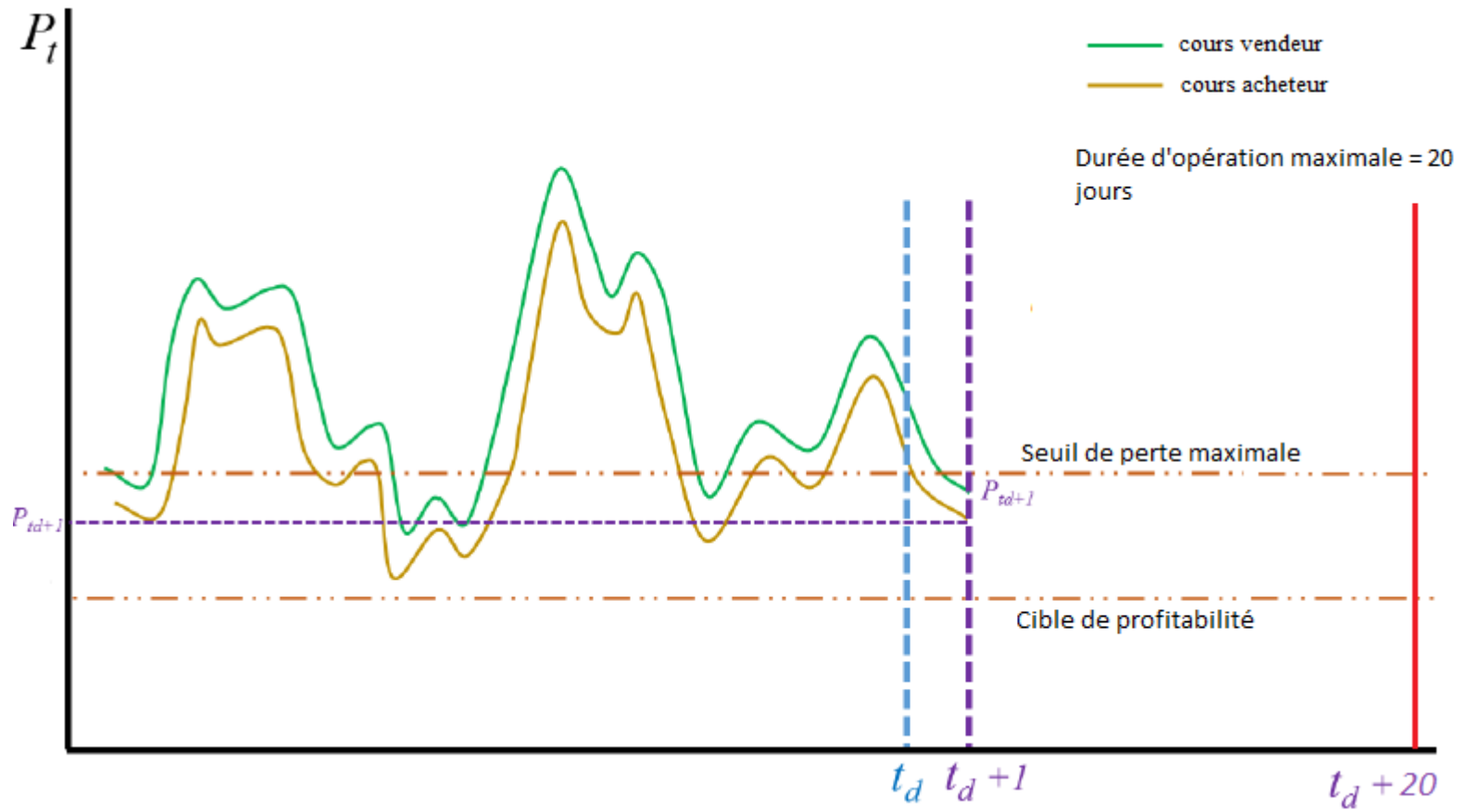
Figure A.4 Mécanisme de transaction sur les marchés
