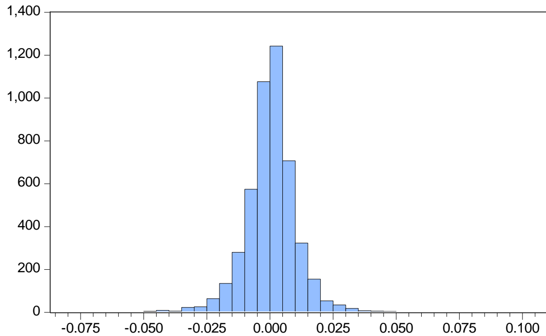
Figure A.1 Distribution des rendements de l'indice de référence
