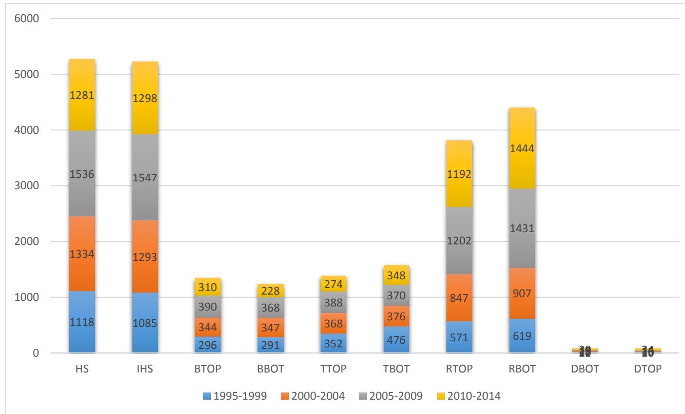
Figure A.5 Fréquence de détection des configurations apparentes par sous-échantillon
