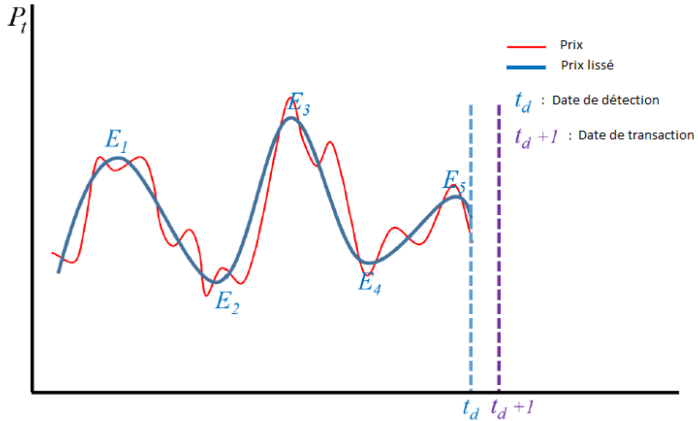
Figure A.3 Lissage des prix par une régression locale polynomiale
