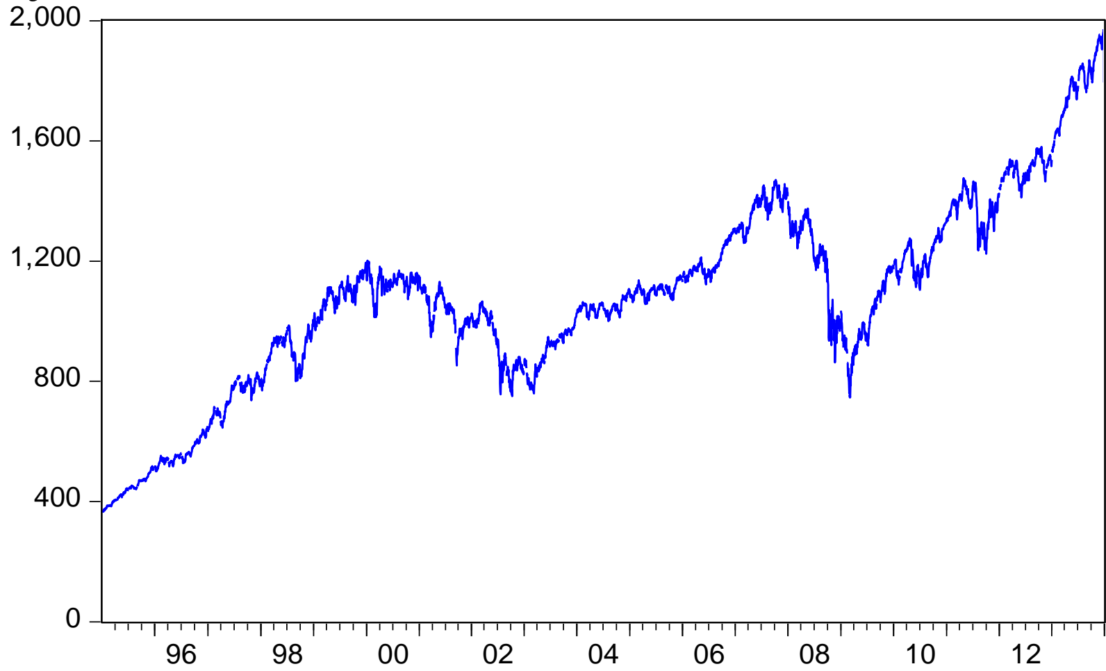
Figure A.2 Evolution de l'indice de référence
