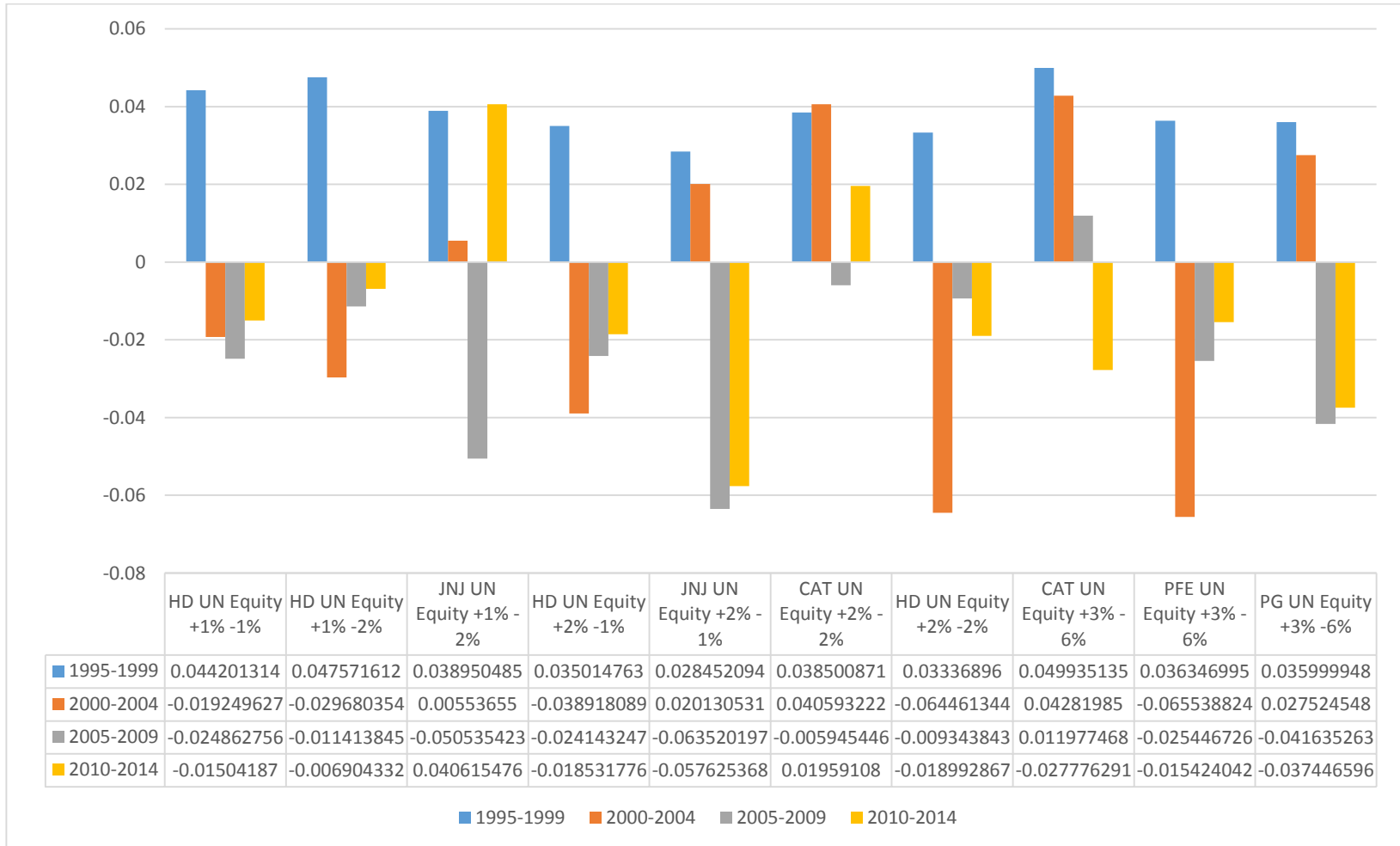
Figure A.7 Ratio de Sharpe pour les stratégies sélectionnées
