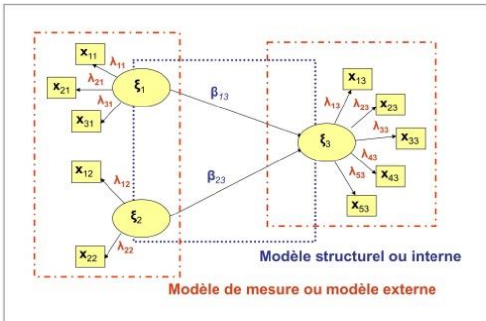
Figure 3.2 Diagramme complet du modèle d'équations structurelles
